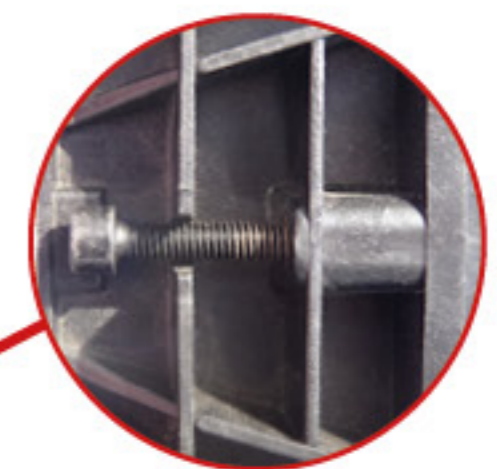
Tapa bloqueable gracias a una llave específica (6 pan). Sistema disimulado debajo de la tapa.
